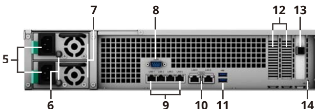
Задняя панель
